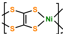
図 1. poly(NiETT)の化学構造
