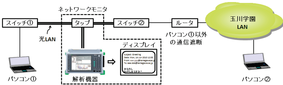
図1：ネットワークモニタ実験の構成
