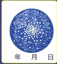
M15 ペガスス座の球状星団
