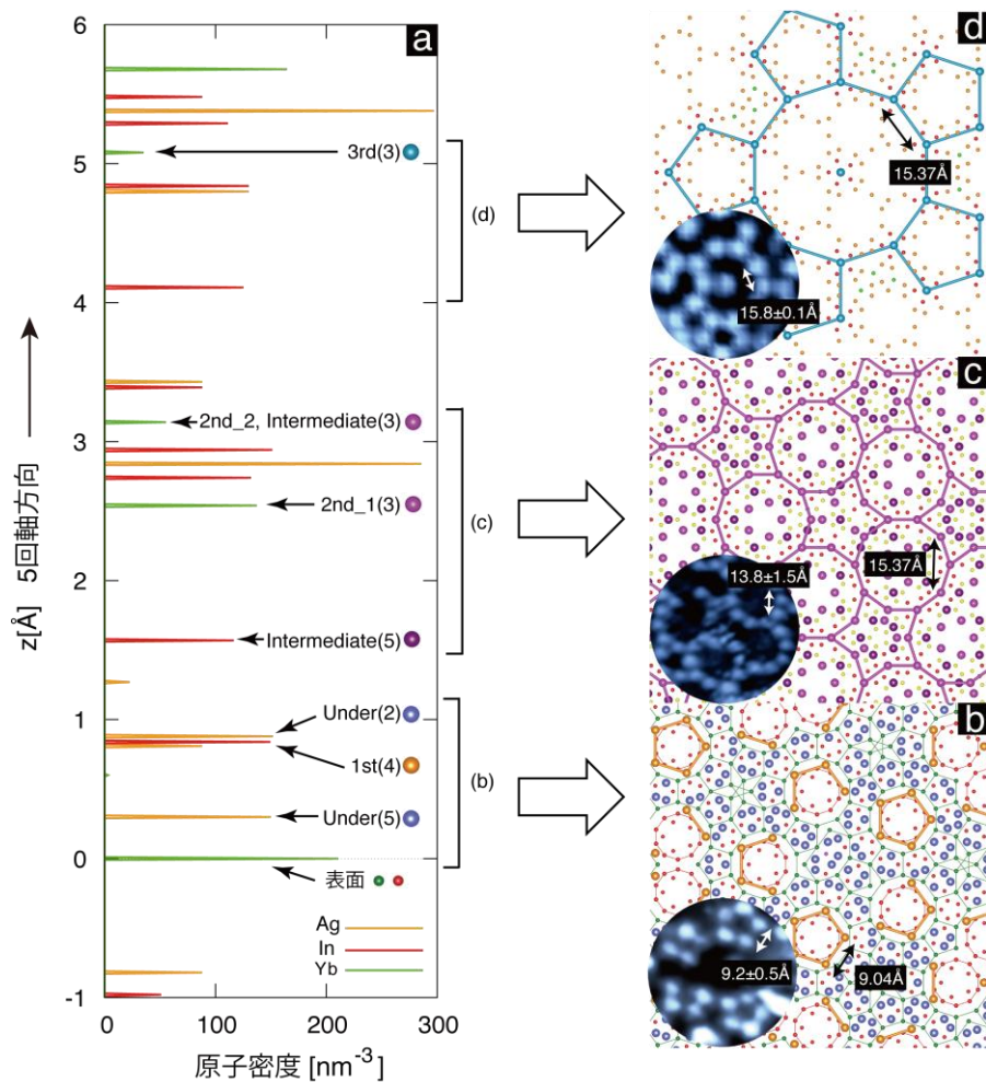
図3(a): 準結晶構造データから求めた基板表面(5回回転対称表面)に垂直な方向の原子密度分布。ここで、Å(オングストローム)は長さの単位で、 1\text{\AA}=10^{-10}\text{m}=0.1\text{nm} (ナノメートル)。 z=0 が表面原子層。図中の矢印は実験で観測された計6原子層(表面に近い側から under層、第1層、中間層1、第2層、中間層2、第3層)に対応する原子層。カッコ内の数字は図2のクラスタの殻番号。(b-d): 表面から(b) 0\leq z\leq 0.9\text{\AA} , (c) 1.53\text{\AA}\leq z\leq 3.15\text{\AA} , (d) 5.04\text{\AA}\leq z\leq 5.40\text{\AA} の範囲の原子位置と鉛の吸着量に応じて観測されたSTM像(挿入図)。それぞれのSTM像と同じ五角形や十角形が基板準結晶の構造データの中にあることが分かる。
