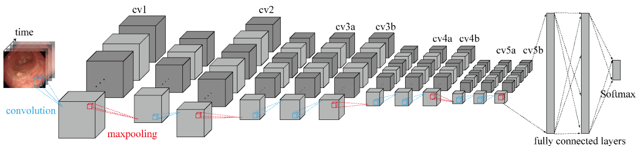
図 1. 3次元畳み込みニューラルネットワーク
