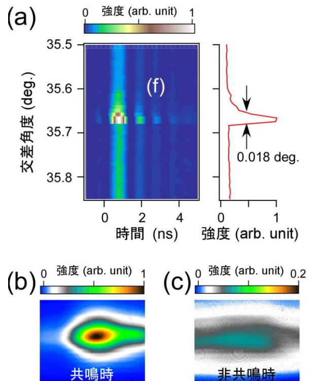
図2 (a) 超蛍光の強度をオシロスコープの時間（横軸）、励起ビームの交差角度（縦軸）に対してプロットした実験結果。1 ナノ秒近辺のピーク領域に関して積分した結果を図の右側に表示している。共鳴条件下 (b) と非共鳴条件下 (c) において測定された超蛍光のビームプロファイル
