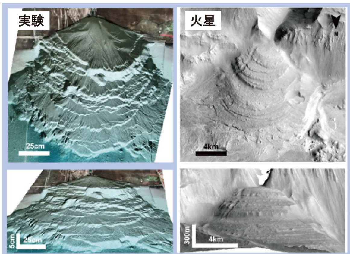
図3 閉鎖湖内の水位上昇で形成されたデルタ（ステップデルタ）とその火星類似地形。
